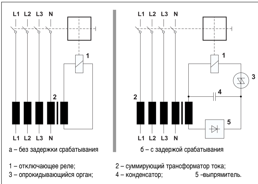
Риц. 17 Структурные схемы УЗО
