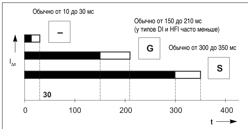
Риц. 31 Обычные значения времени отключения УЗО при испытании дифференциальным током, равным I_{\Delta n}
