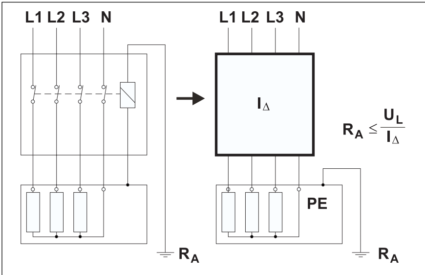
Риц. 34 Замена УЗО типа FU на УЗО, управляемое дифференциальным током
