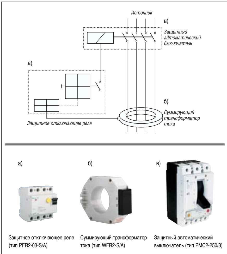
Рис. 13 Структурная схема УЗО с непрямым отключением
