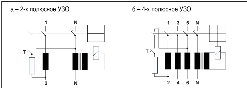
Рис. 14 Структурные схемы УЗО с различным числом полюсов
