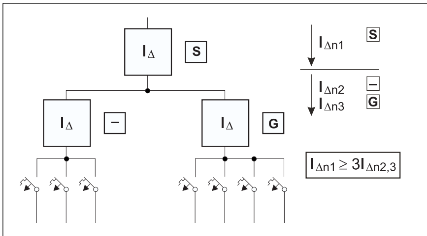
Риц. 20 Схема участка сети с селективно работающими УЗО
