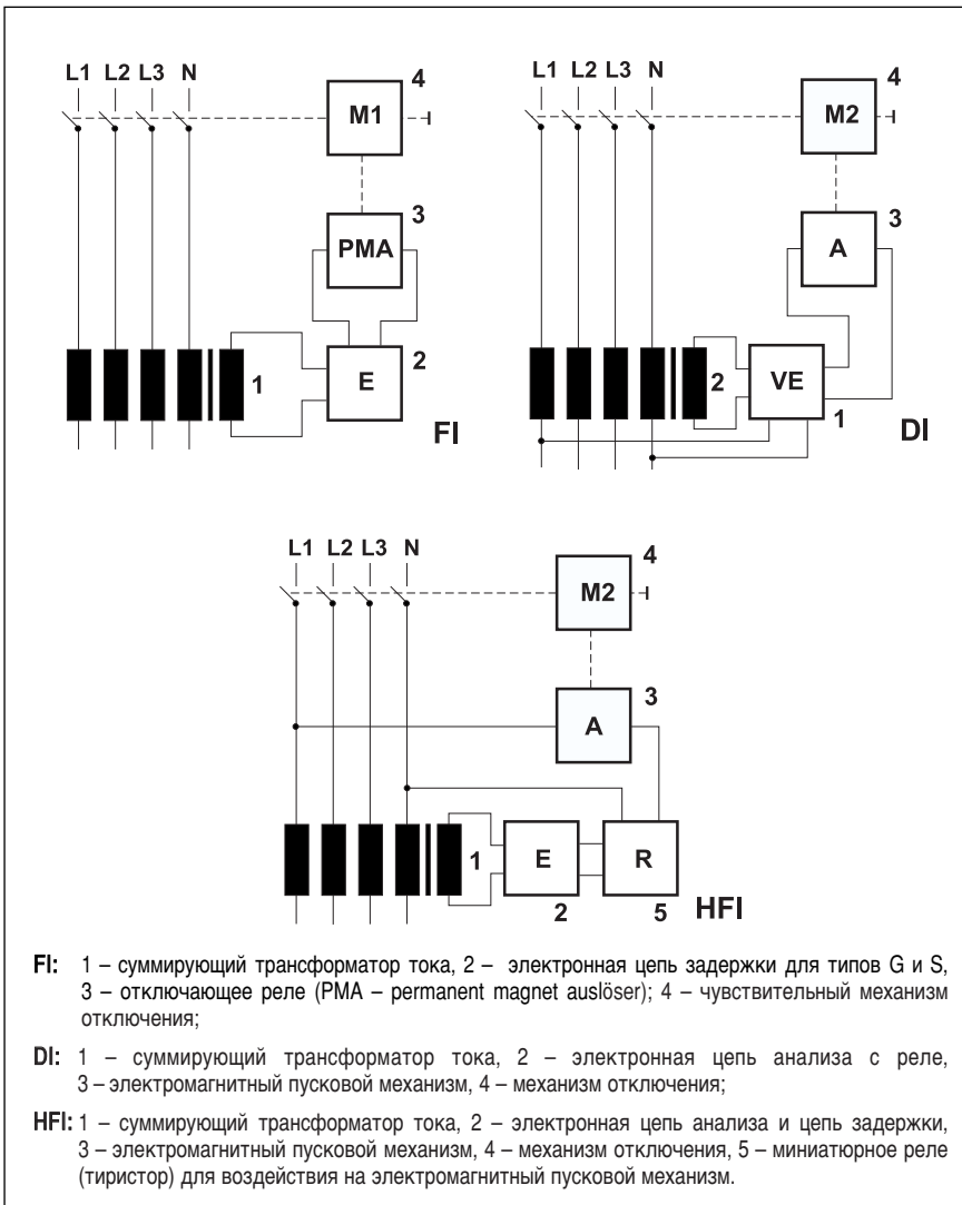
Рис. 16 Структурные схемы УЗО типов FI, DI и HFI
