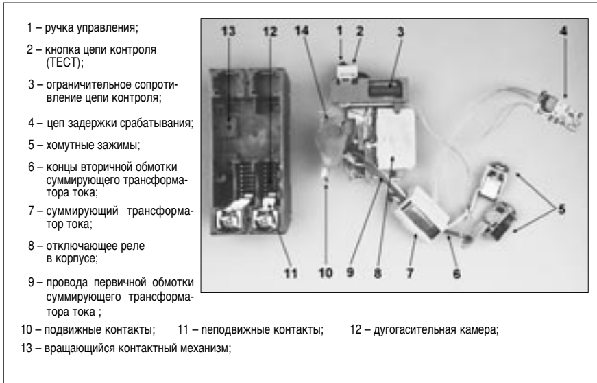
Риц. 18 УЗО с задержкой срабатывания (типы G и S)
