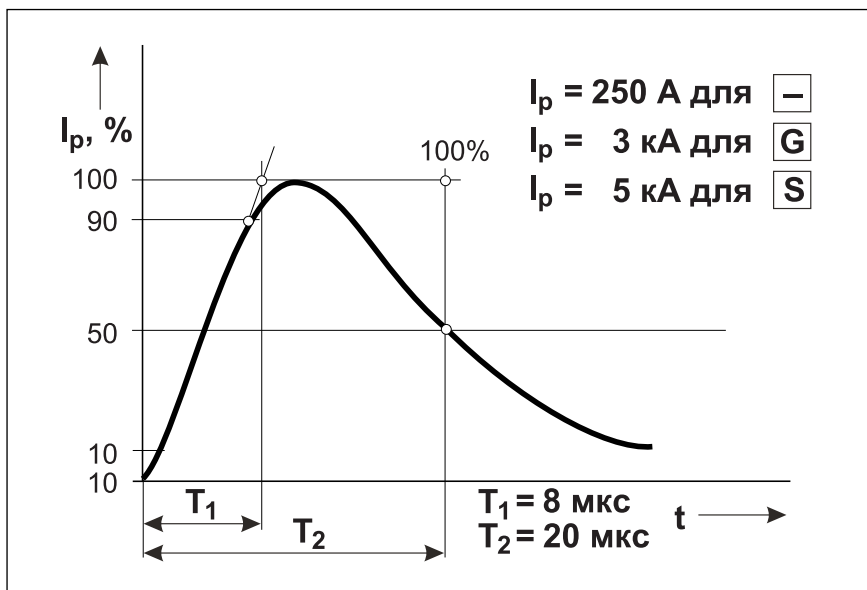
Рис. 40 Нормализованная форма ударной волны тока 8/20 мкс 1)
