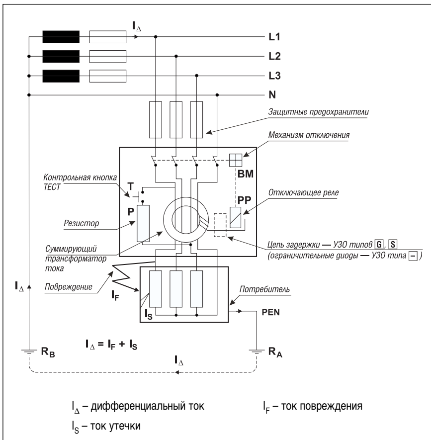
Рис. 10 Принципиальная схема подключения УЗО (сеть системы ТТ)
