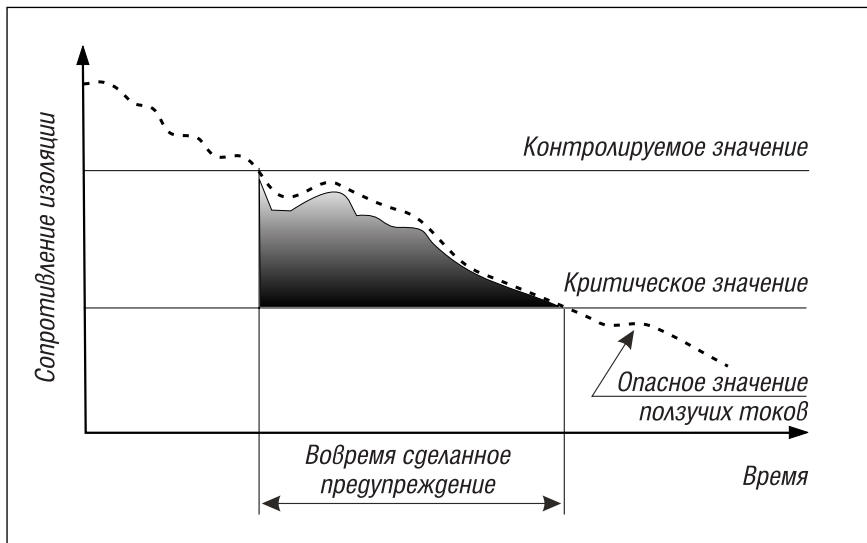
Риц. 27 Изменение состояния изоляции электропроводок и оборудования в результате старения изоляции
