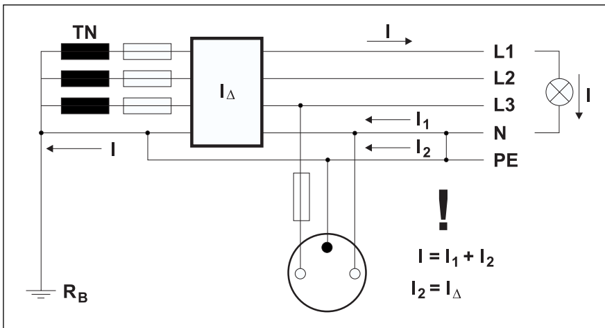
Рис. 35 Недопустимые соединения проводников PE и N за УЗО
