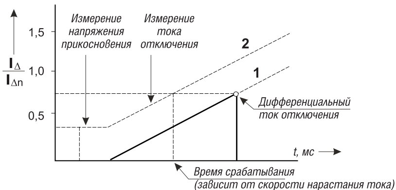
Риц. 30 Зависимости нарастания значения тока от времени при определении минимального отключающего дифференциального тока УЗО
